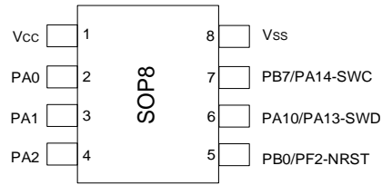
图 3-13 SOP8 PY32F003L2xSx (Top view)
